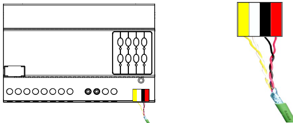
HDL-Buspro Wiring Diagram
