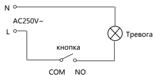
Рис 6. Подключение
