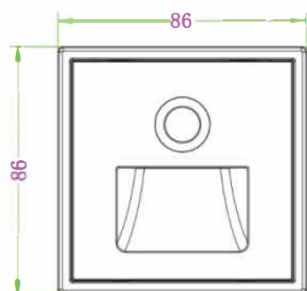
Рис 2. Размеры – Вид спереди Пластиковая рамка
