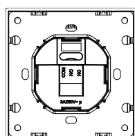
Рис 5. Вид сзади
