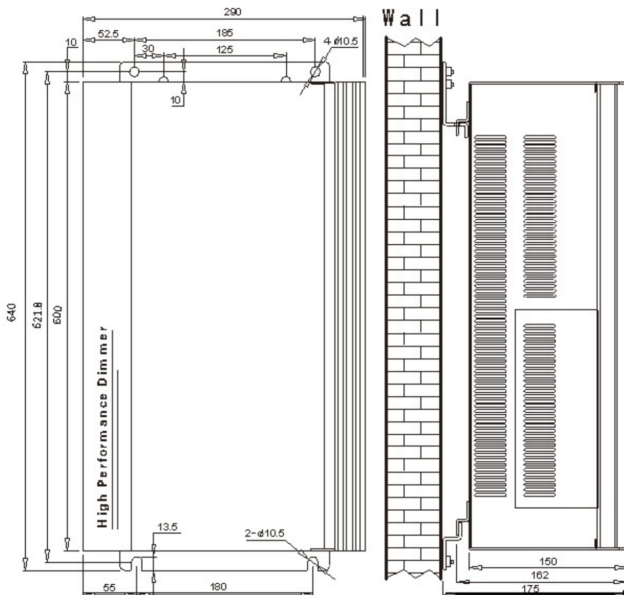
Габариты установки
