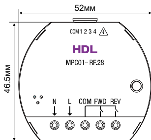
Рис 2. Габариты - Вид спереди
