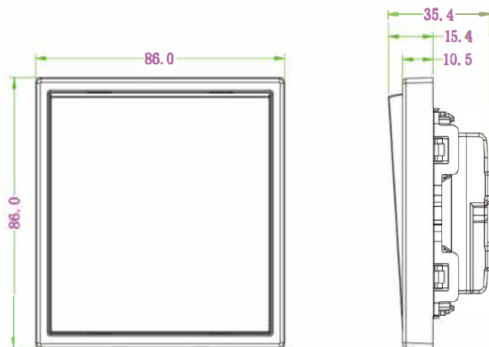
Рис. 2. Размеры - Вид Спереди сбоку
