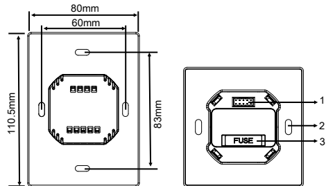
Рис. 5. Габариты - Вид сзади
