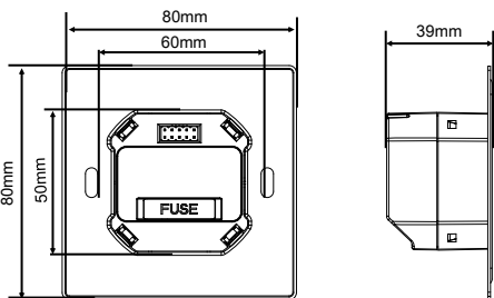
Рис. 3. Габариты - Вид спереди
