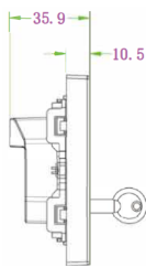
Рис 4. Размеры – Вид сбоку
