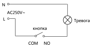
Рис 6. Подключение
