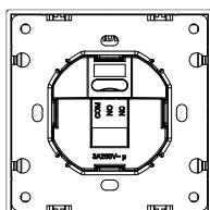
Рис 5. Вид сзади
