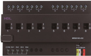
Рис 2. DIN Реле, 8-канальное, 16А на канал с сухими контактами
