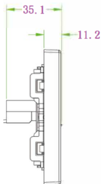
Рис 3. Размеры - Вид Сбоку
