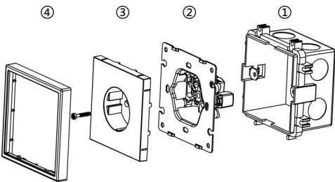
Рис 5. Установка
