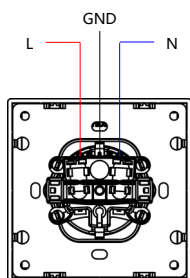
Рис 4. Подключения
