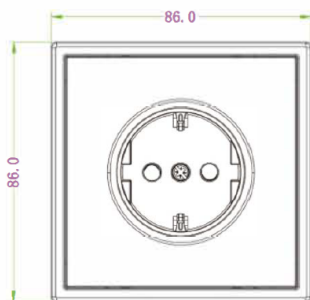
Рис 2. Размеры - Вид Спереди
